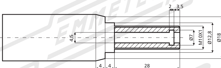
Schema di filettatura Threading scheme
