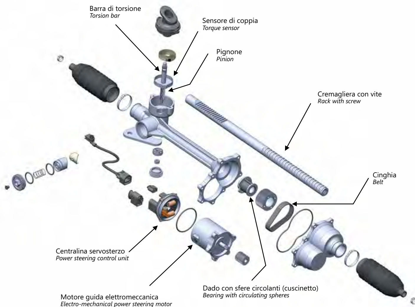
Cremagliera elettromeccanica Electric-mechanical rack
